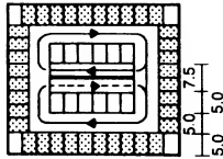
2 Longitudinal ramp
